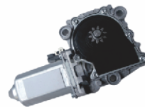
MTP 400026 - 3176550 Motor Vidro Elétrico volvo LD MTP 400025 - 3176549 Motor Vidro Elétrico Volvo LE
