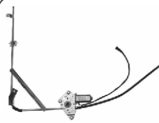
MTP 325717 - 2997195 LD MTP 325718 - 2997196 LE Máquina Vidro Elétrico C/ Motor Stralis LD / LE
