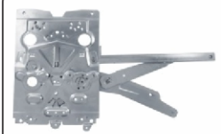
MTP 400147 - 3176546 Maq. Vidro Elétrico S/Motor LD MTP 400148 - 3176545 Maq. Vidro Elétrico S/Motor LE
